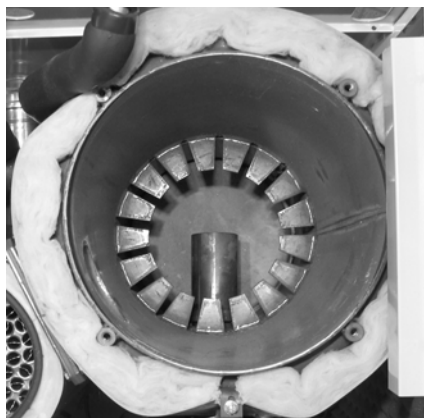
Giri dei fumi STRATON 17 / 21
